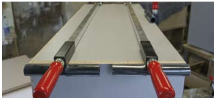
Verleimen von Schränken, Korpussen, gedübelt oder mit Flachdübel Glueing of cabinets, corpuses, dowelled drawers, laminated drawers
